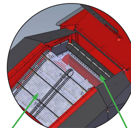
Option chaîne intervalle 11mm Option égalisateur de trémie
